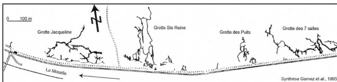
Figure 3 : Plan d'ensemble des grottes de Pierre-la-Treiche. Toutes les grottes situées en rive droite de la Moselle, en amont de Toul contiennent des alluvions d'origine vosgienne (galets de quartz notamment) qui montrent que ces cavités souterraines ont servi de perte karstique pour les eaux de la Moselle.
