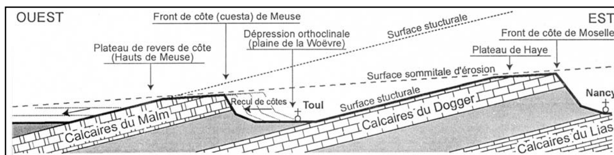
Figure 1 : Coupe géologique schématique de la Meuse à la Meurthe, passant par Toul et Nancy. Noter les deux fronts de côtes (de Meuse et de Moselle), correspondant aux deux grandes masses calcaires du Dogger et du Malm. Noter aussi la surface d'érosion recoupant à l'emporte-pièce l'ensemble des reliefs de la Lorraine sédimentaire.
