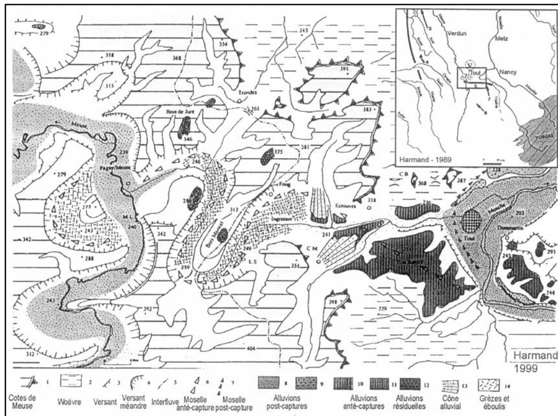
Figure 2 : Le site de capture de la Moselle aux alentours de Toul. Noter le coude de capture de la Moselle qui se dirige à présent vers le nord-est. Le Val de l'âne, parcouru actuellement par l'Ingressin correspond à l'ancien couloir de la Moselle lorsqu'elle se dirigeait encore vers la Meuse. Il ne reste de ce passage qu'une forme de vallée bien marquée et des alluvions anciennes, d'origine vosgienne, recouvertes aujourd'hui d'un tablier d'éboulis calcaire.
