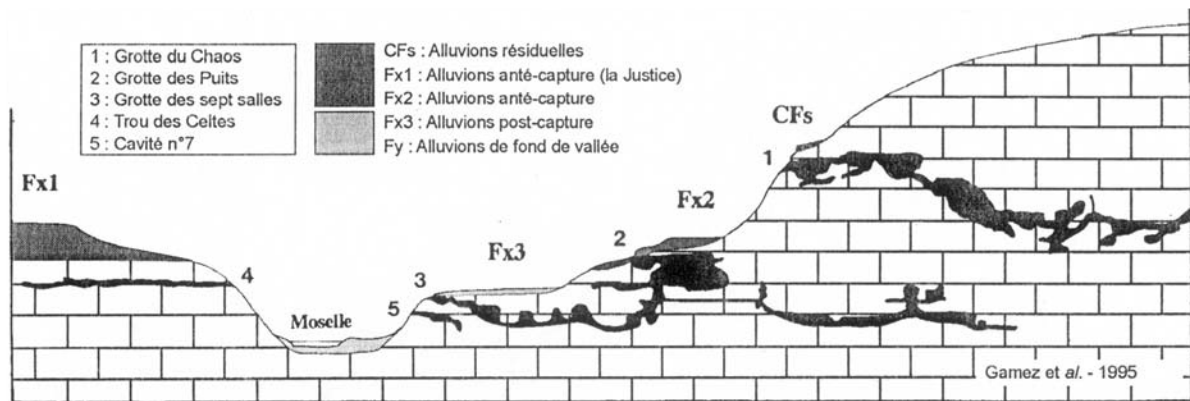
Figure 4 : Relations entre les cavités du karst et les terrasses alluviales de la Moselle au niveau de Pierre-la-Treiche. Toutes les grottes connues s'étagent sous des terrasses et se sont mises en place avant la capture de la Moselle. Les eaux de la Moselle perdues dans le karst, lors de cette mise en place, pouvaient alimenter la vallée de la Meurthe et participer ainsi à la capture de la Moselle.
